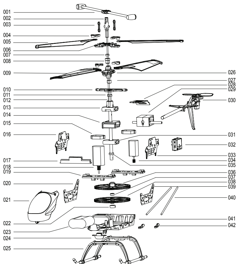
遥控直升机分解图
