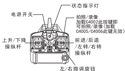
遥控器
