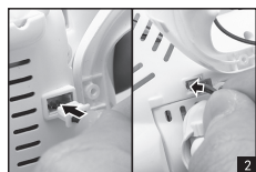
2. 将摄像头连接线的白色接口跟摄像头上的接口连接，再将摄像头连接线的红色接口插入下主体上的C4006接口上。
