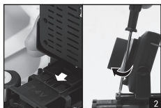
2. 将摄像头扣在电池座的扣位上, 再将螺丝按顺时针旋转扭紧。
